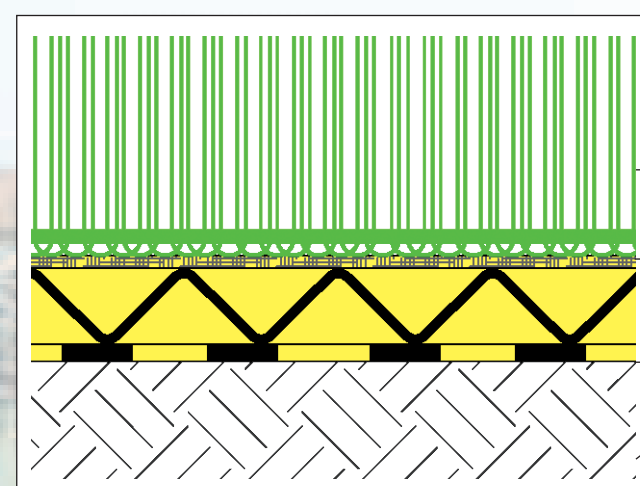
VÍZSZINTES VÍZELVEZETÉSI MEGOLDÁS GEODRÉN ÉS TÖMÖRÍTETT TALAJ METSZETE
